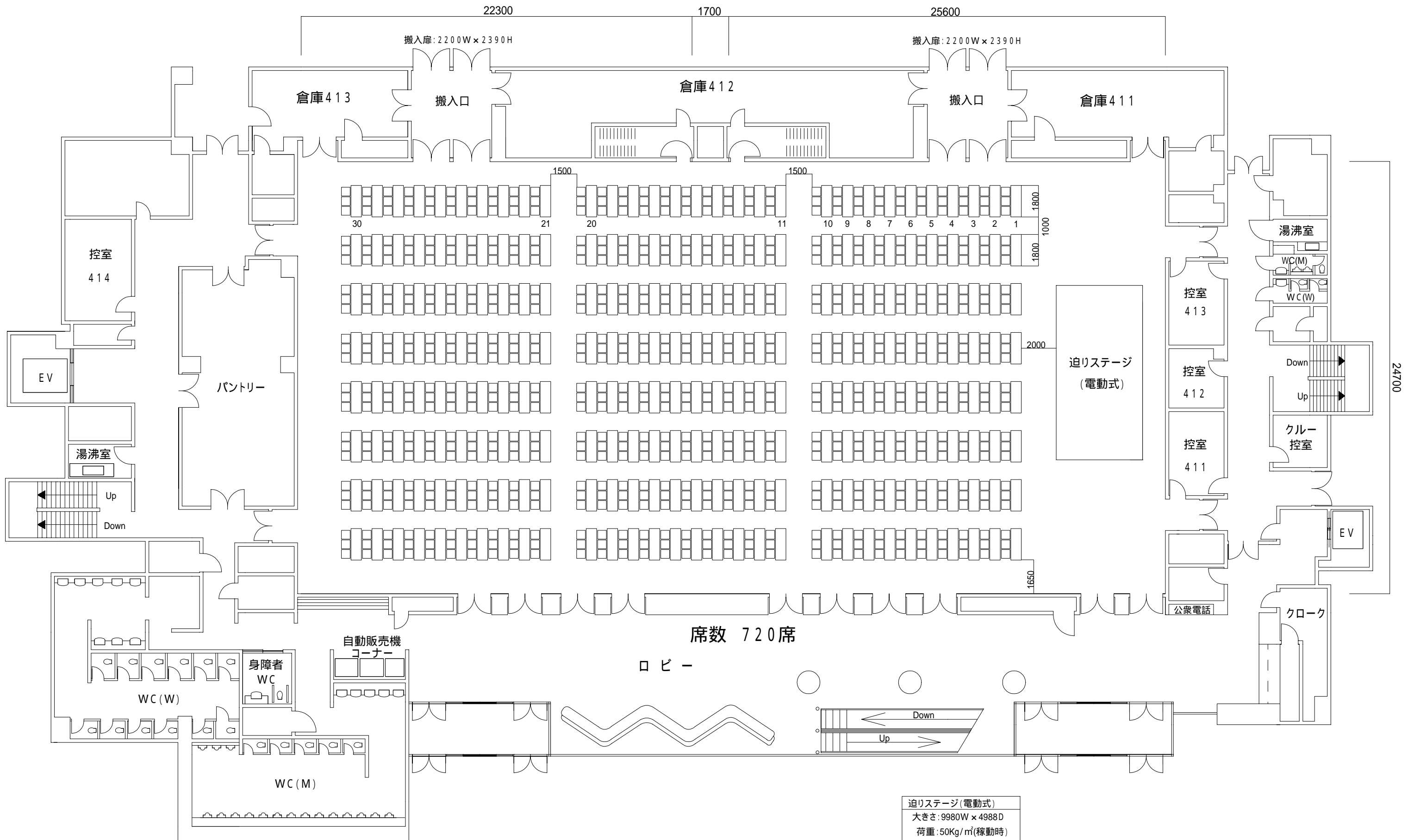
白鳥ホール 平面図
