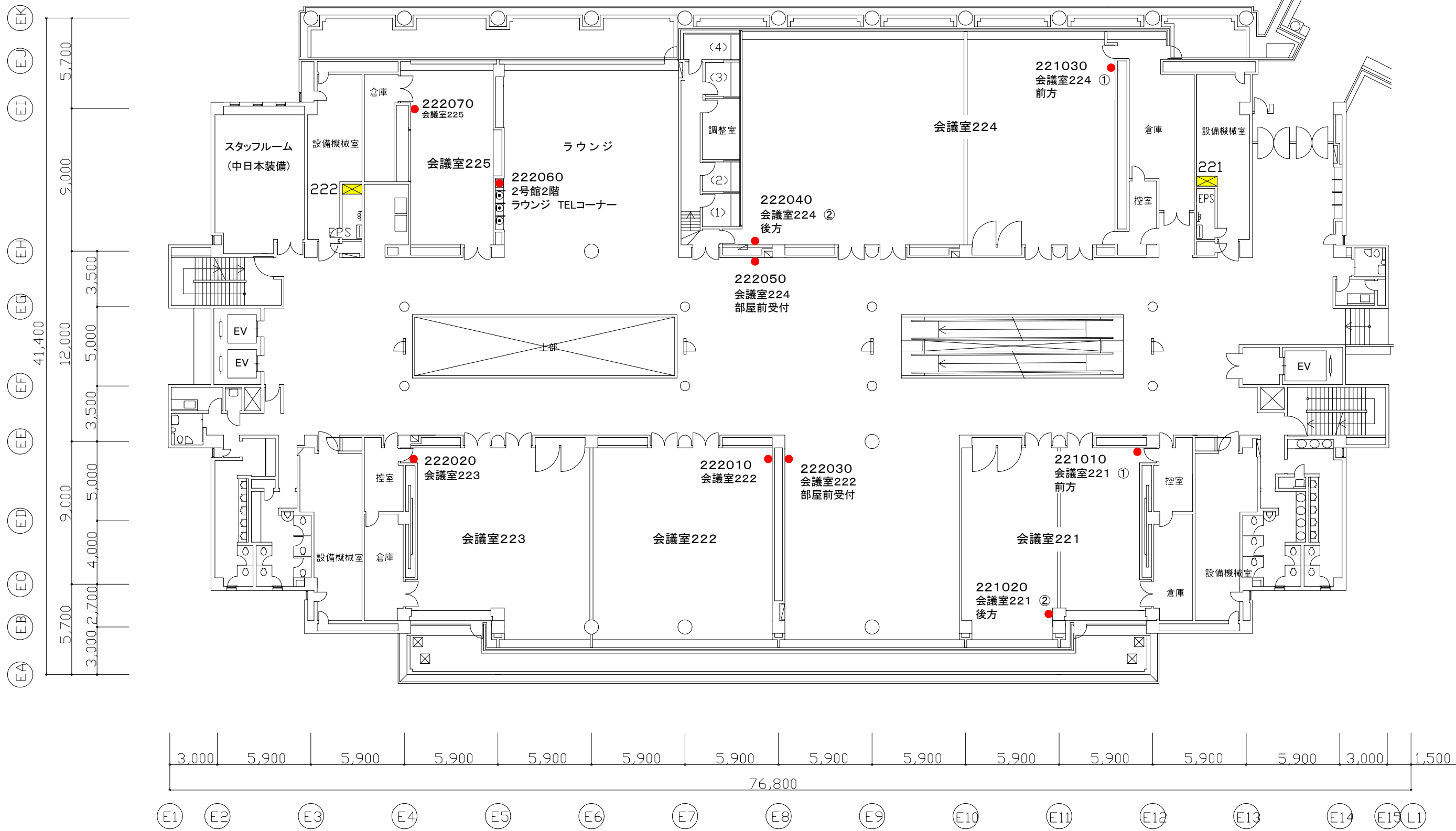
2号館2階平面図 情報コンセント配置図
